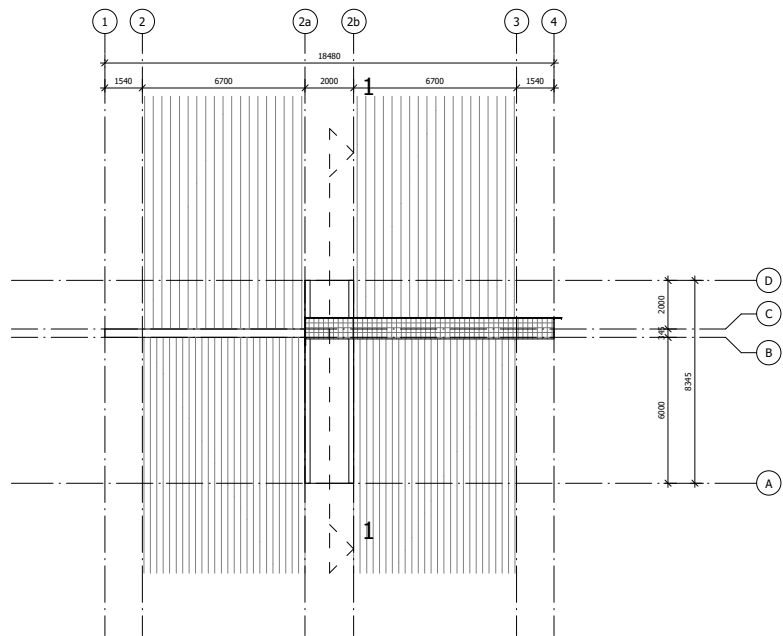
Bovenaanzicht: schaal 1:100
