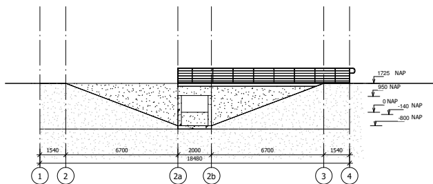
Dwarsdoorsnede: schaal 1:100
