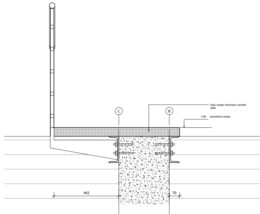
Detail 02 : schaal 1:5
